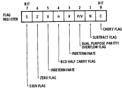
Fig. 2-6. Flag register format.
