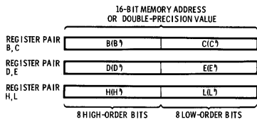
Fig. 2-4. Register pairs.
