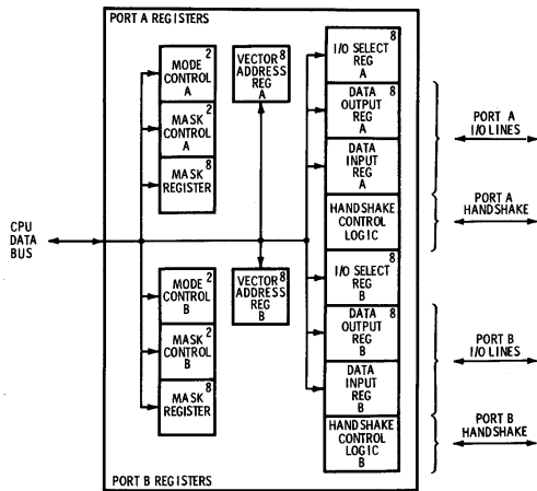
Fig. 8-7. PIO registers.
