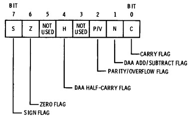
Fig. 6-1. Flag register format.
