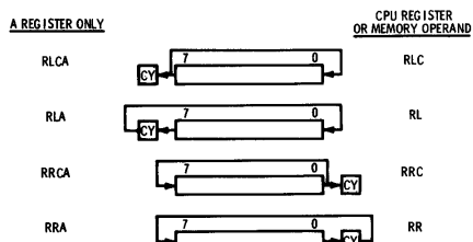
Fig. 12-2. Shift actions.
